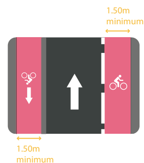
Aménagement d'une piste cyclable en « contresens » en cas de trafic motorisé supérieur à 4 000 véhicules/jour
