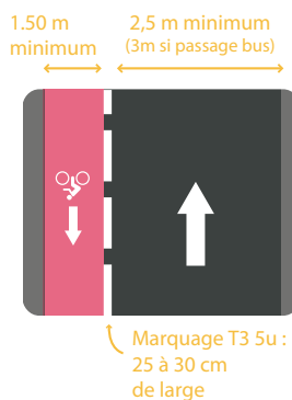
Aménagement classique d'un double-sens cyclable
