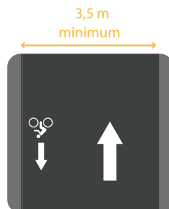
En cas de contrainte de largeur, marquage via pictogramme en section courante
